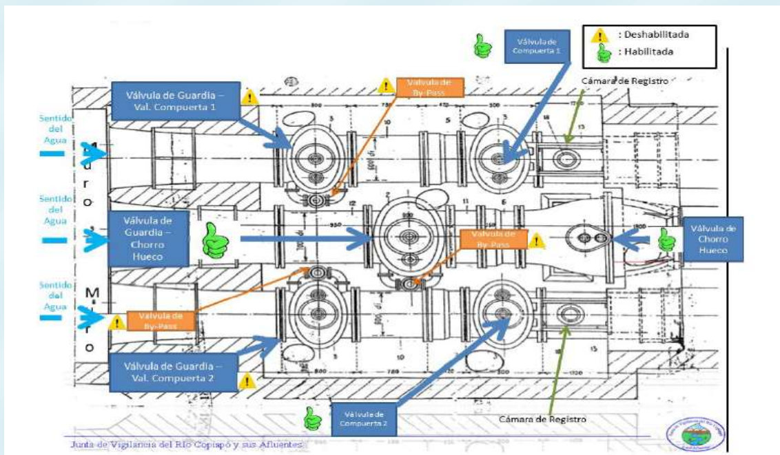
Esquema de válvulas Lautaro
